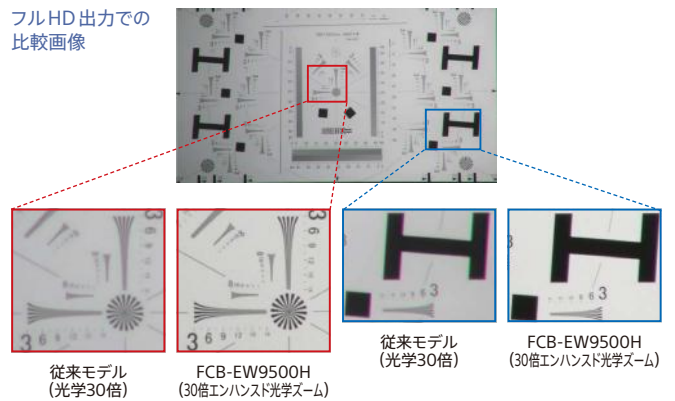
0.03lx Halogen 1/30s ICR:ON HS:OFF時の比較画像
