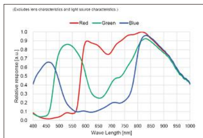
分光感度特性
